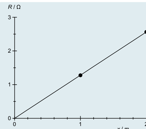
Fig. 4 Résistance R en fonction de la longueur
