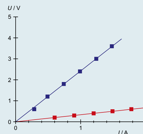
Fig. 1 Diagramme tension/courant ( U-I ) pour un fil en constantan (bleu) et un fil en laiton (rouge)
