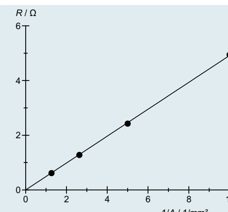
Fig. 5 Résistance R en fonction de l'inverse de la section transversale A
