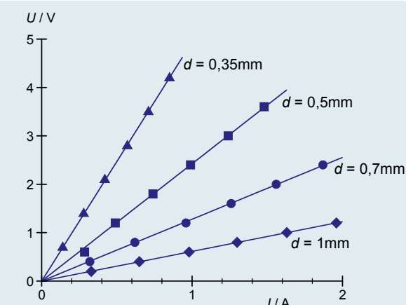
Fig. 3 Diagramme tension/courant ( U-I ) pour des fils en constantan de différentes épaisseurs
