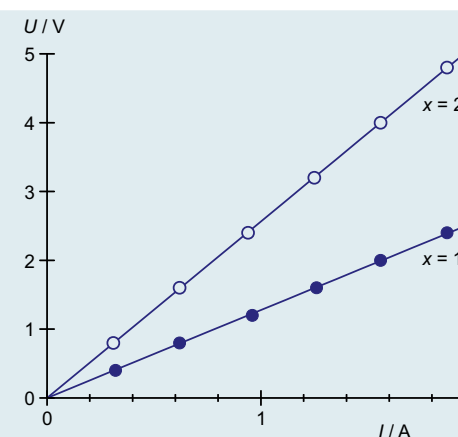
Fig. 2 Diagramme tension/courant ( U-I ) pour des fils en constantan de différentes longueurs
