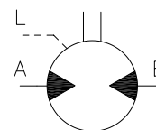
SAI9436 - Moteur à pistons axiaux
