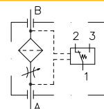
SAI9462 - Filtre de pression avec indicateur de colmatage
